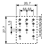
Csatlakozók nézetjei
