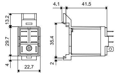
056.27 relével
