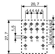
Csatlakozók nézetjei
