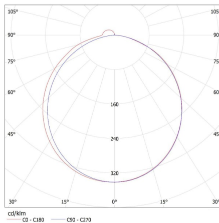
KANLUX S.A. (kat 26680) ASTEN LED IP44-8W-NW / Krzywa rozsyłu światła (biegunowo)
