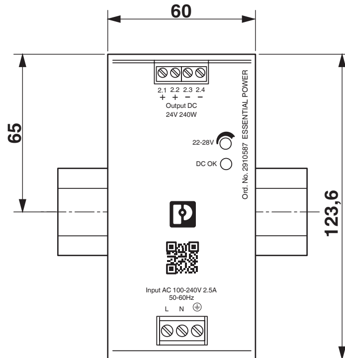
Méretrajz
